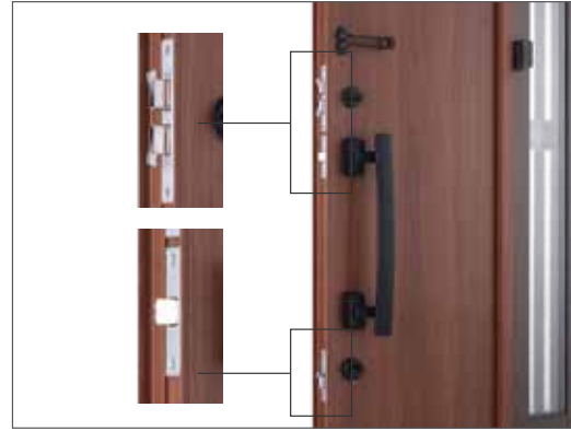
ติดตั้งล็อก 2 จุด ควบคุมกลอนแบบขอเกี่ยว 3 จุด
